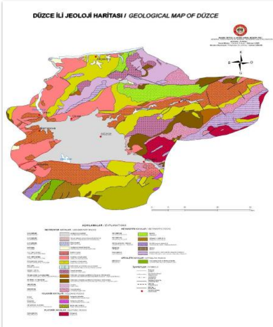
Şekil 3-2 Düzce'nin Jeolojik Haritası
